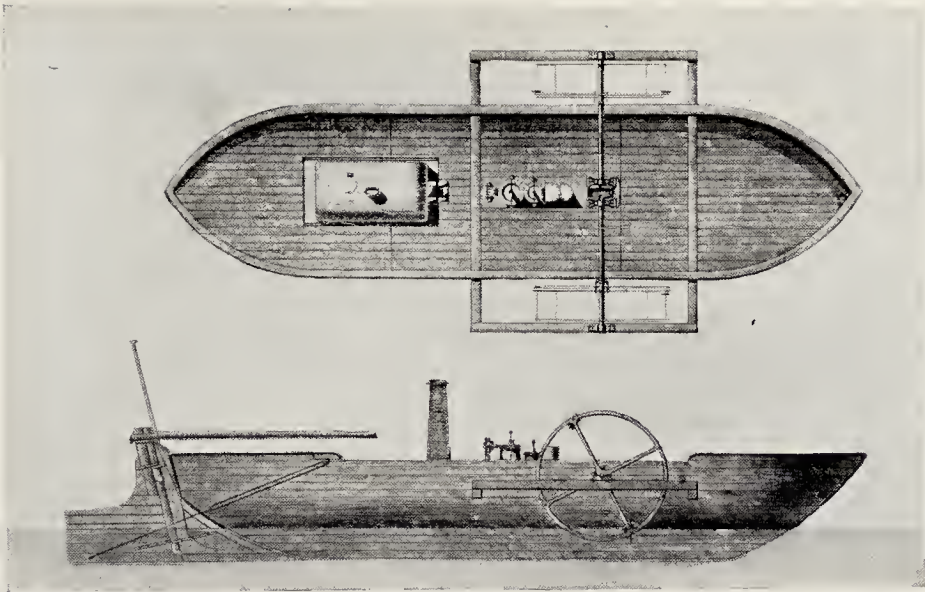
SS. "ELIZABETH" (1815).
